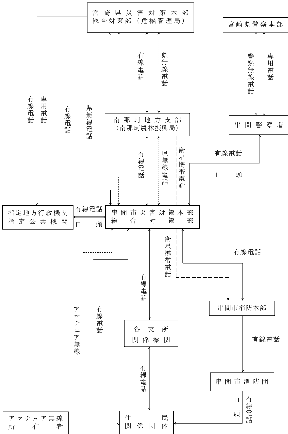
串間市における通信利用系統表
