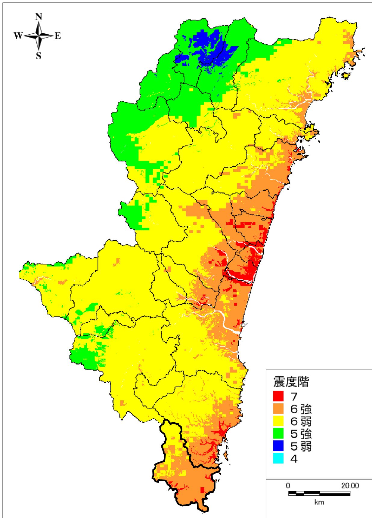
震度分布図
