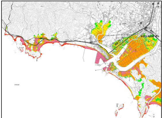
津波浸水深
