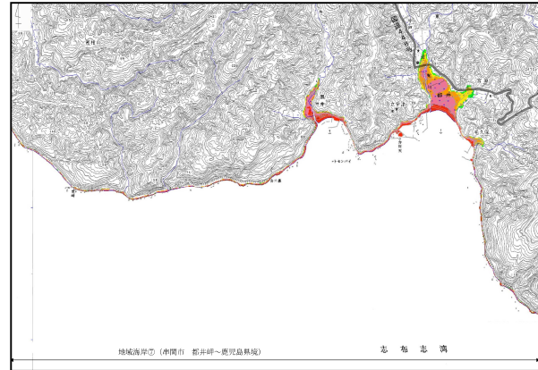
津波浸水深
