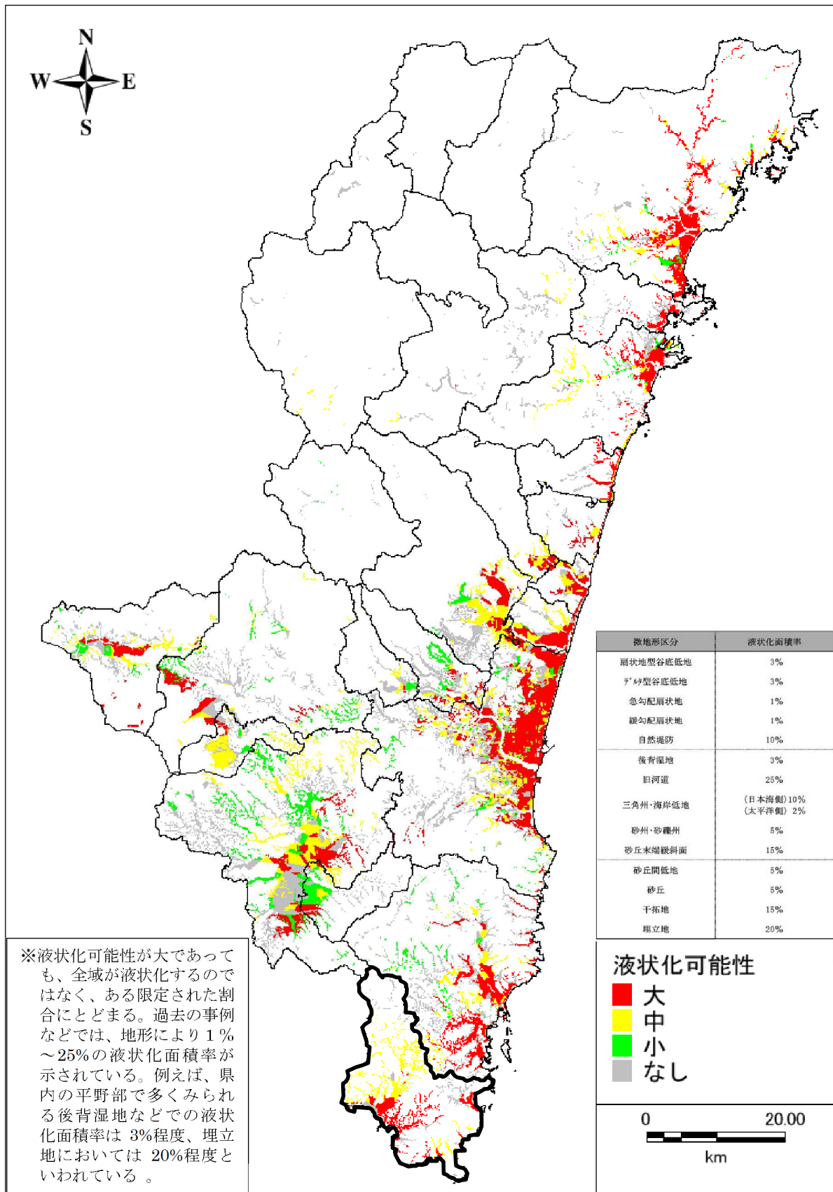
液状化可能性分布図
