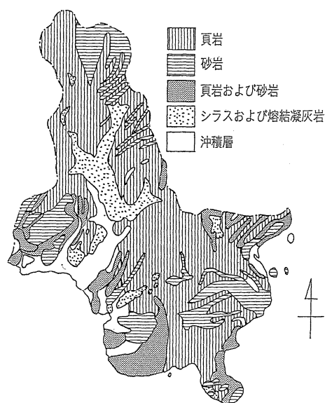
串間市地質図
